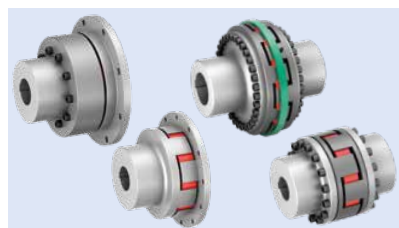
Schwerlastkupplung
