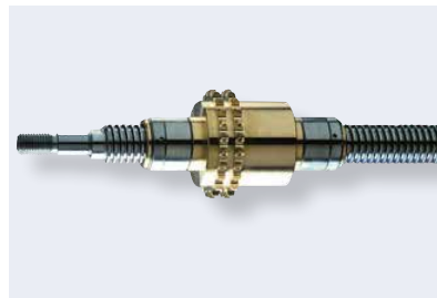
Spindel und Mutter, bearbeitet nach Kundenzeichnung
